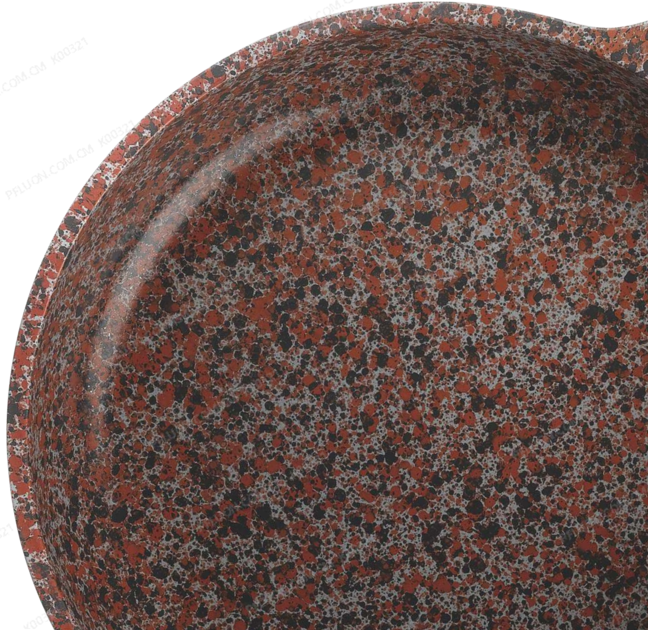
TUNDRA 冻原
